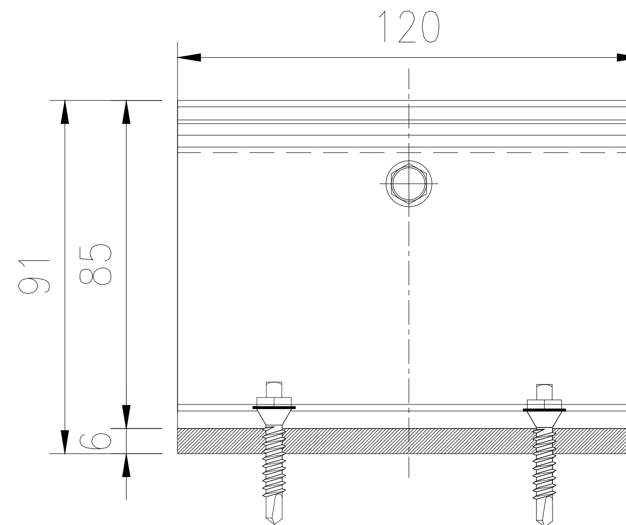
VIEW-D
